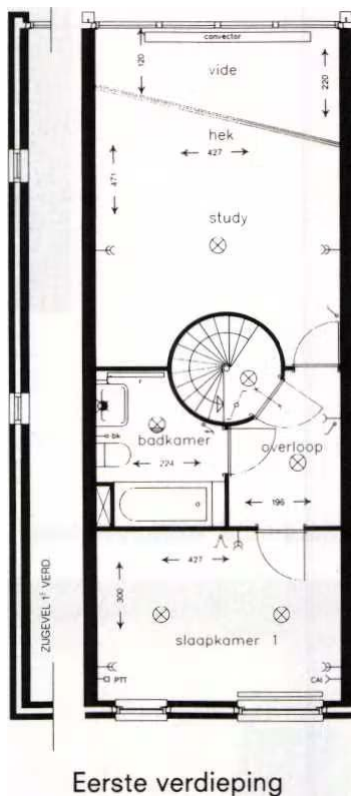
Eerste verdieping
