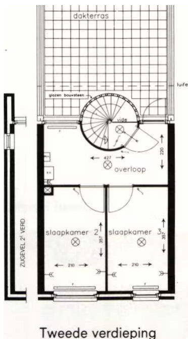
Tweede verdieping
